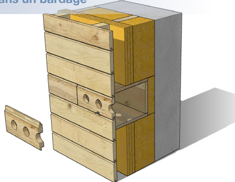
Intégration d'un nichoir dans un bardage
